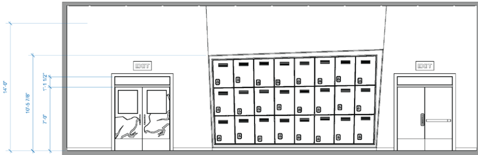
01 SECTION Scale: 1/4" = 1'-0"
