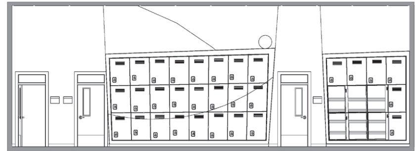
02 SECTION Scale: 1/4" = 1'-0"
